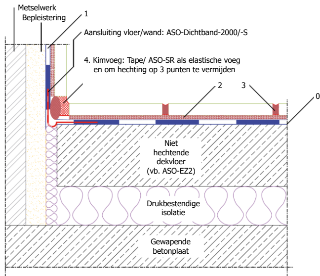
Fig. 3 – Composit-waterdichting onder betegelingen of platen in vochtige ruimten
