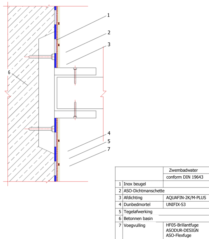
Fig. 11 – Vastzettingflens voor in te voegen stuk
