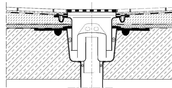
Prevedenie podlahového výpustu (nie je zobrazené v mierke)
