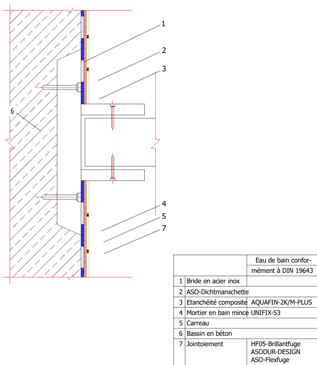
Fig. 11 – Bride de scellement pour pièce à insérer
