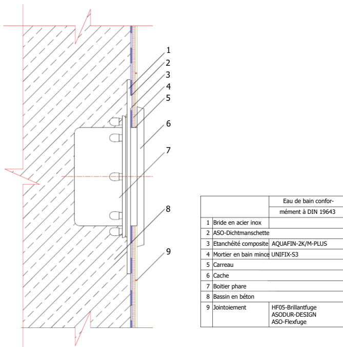
Fig. 10 – Etanchéité de de phares sous-marins avec brides
