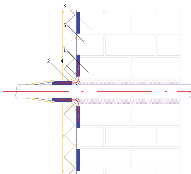
Fig. 3 – Etanchéité composite sous carrelages ou plaques en pièces humides
