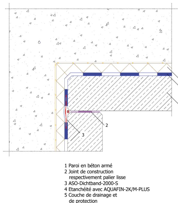
Fig. 2– Etanchéité d'un joint de construction respectivement d'un palier lisse à l'aide d'AQUAFIN-2K/M-PLUS
