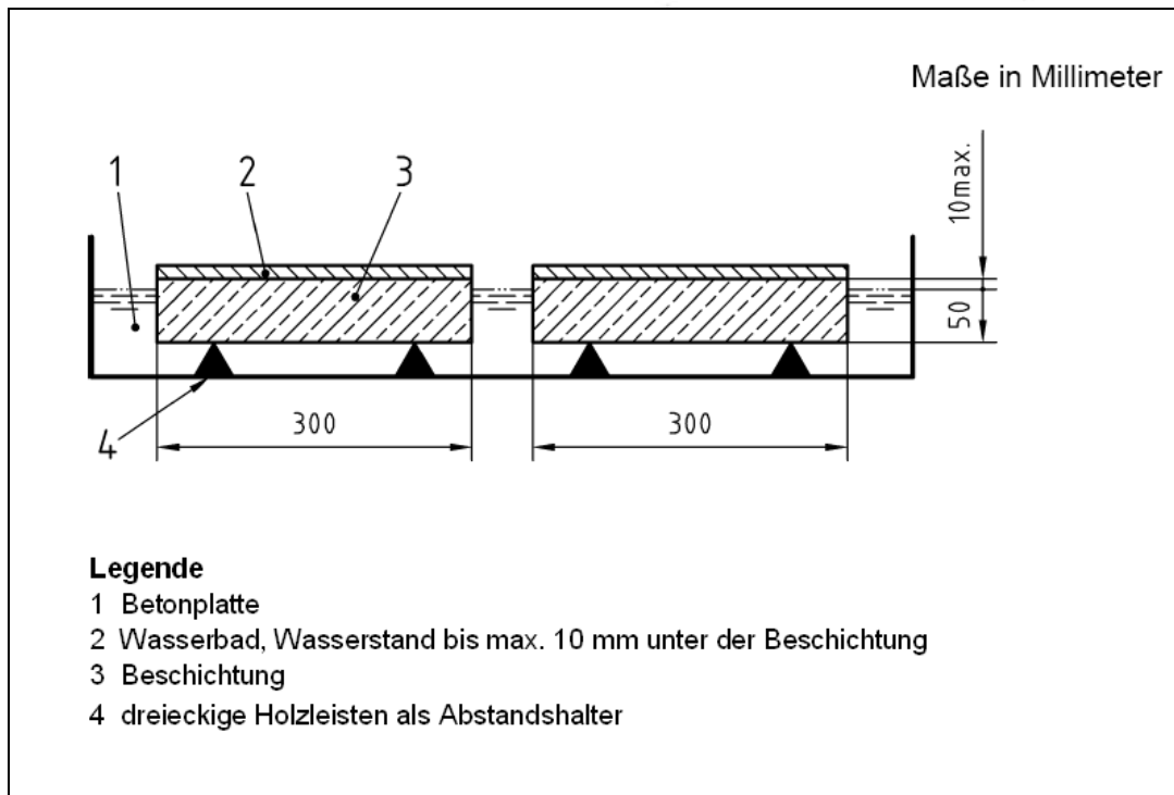
Bild 1: Lagerung der Probekörper im Wasser
